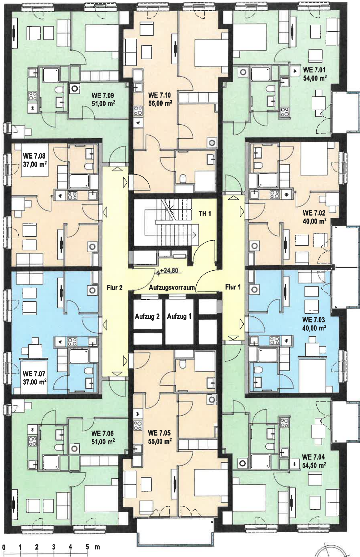
Grundriss 7.OG Wohnen
