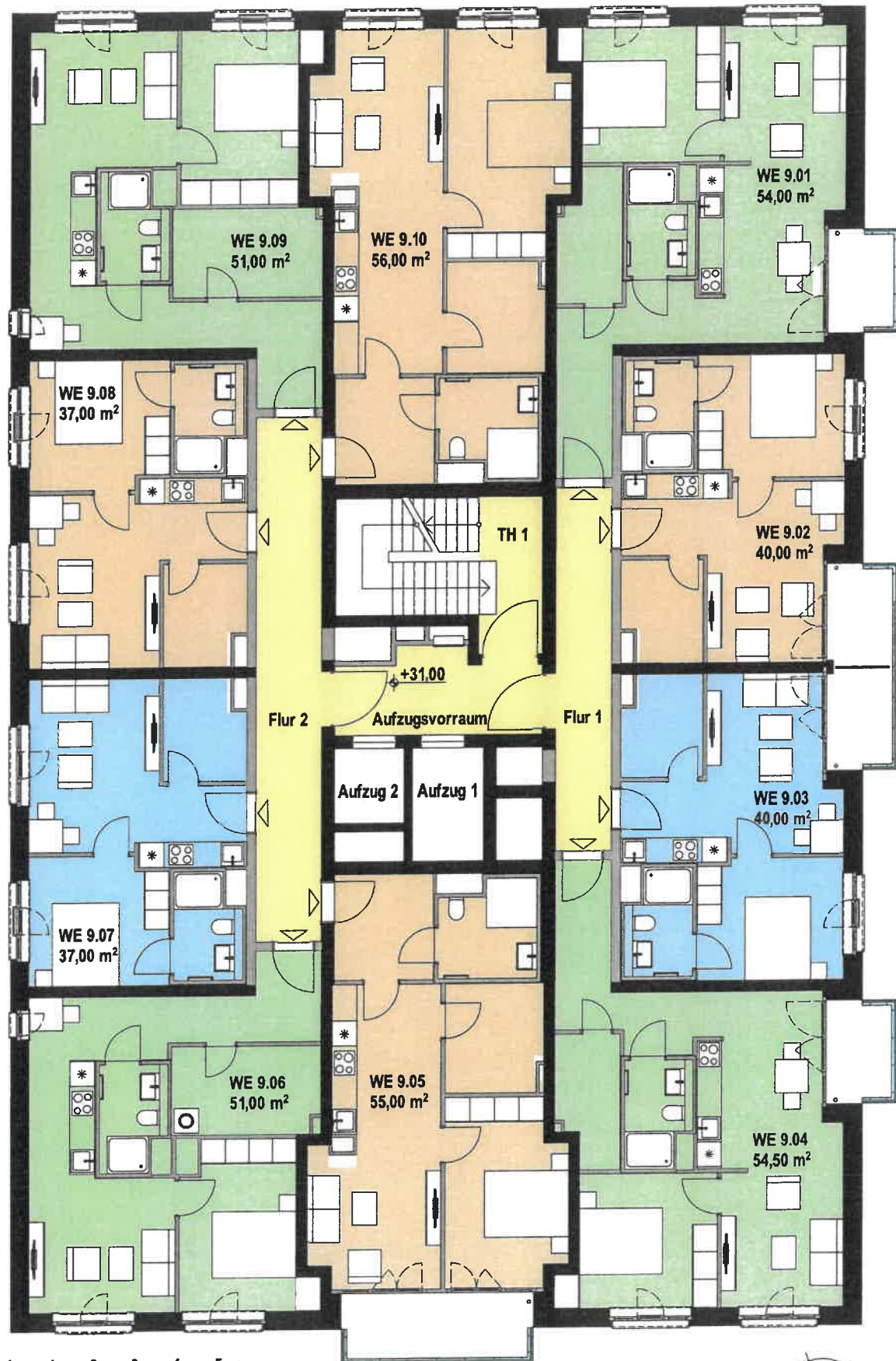
Grundriss 9.OG Wohnen
