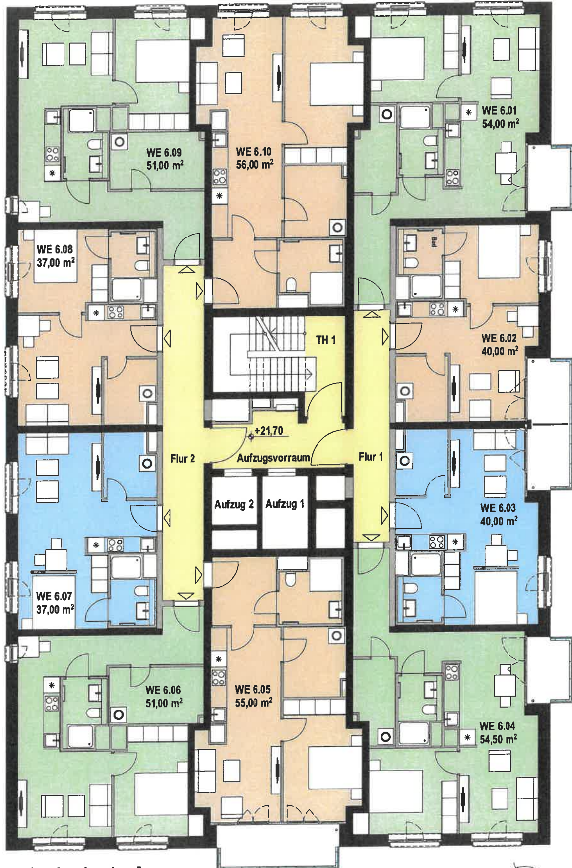
Grundriss 6.OG Wohnen
