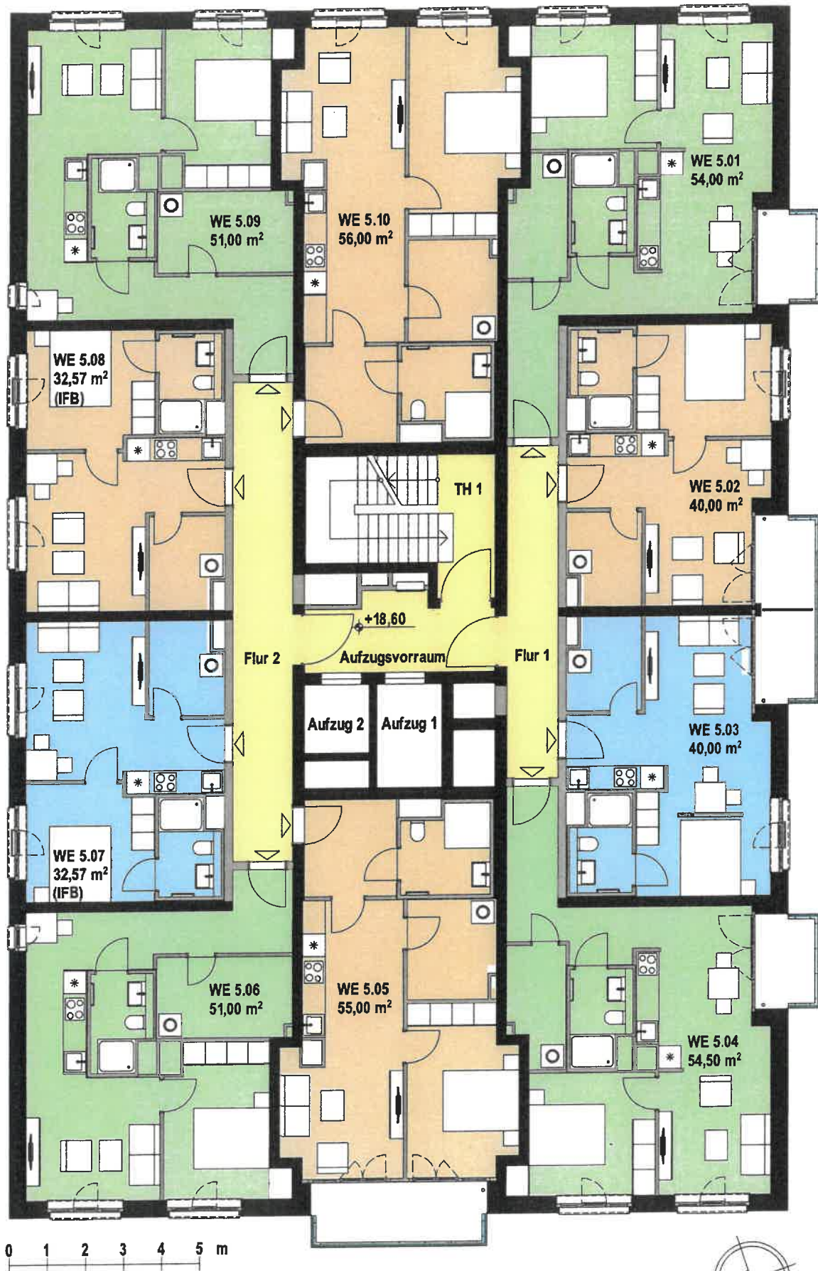
Grundriss 5.OG Wohnen
