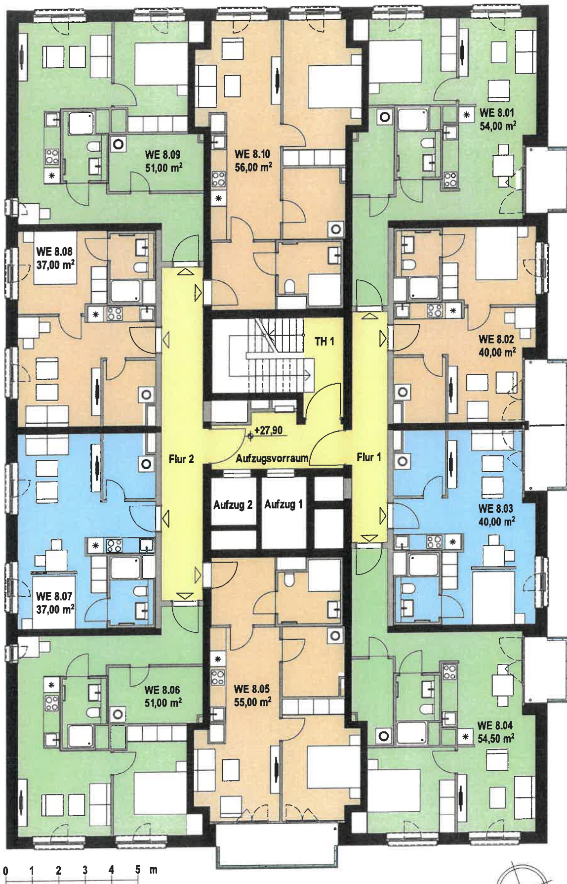
Grundriss 8.OG Wohnen
